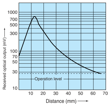
UM2-Z3SV · UM2-Z3DSV
