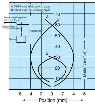
UM2-Z3SV · UM2-Z3DSV
